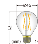
LDG3L-E17/C/24/45/N
