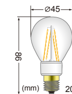
LDG3L-E17/C/24/45/D
