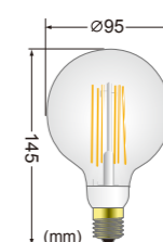
LDG8L/95/D LDG8L/95
