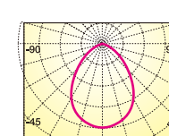
配光曲線
