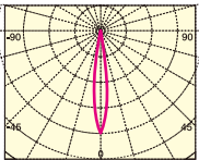
配光曲線
