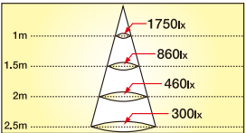
直下照度
