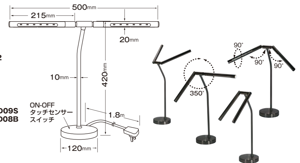
Tバー 寸法図
